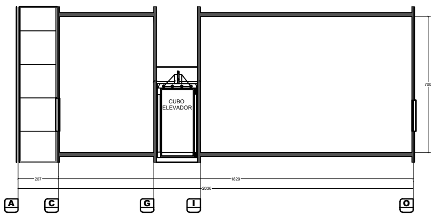
SECCIÓN A-A ESCALA 1:100
